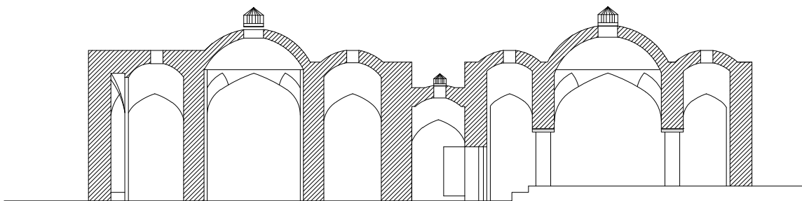
برش B-B
