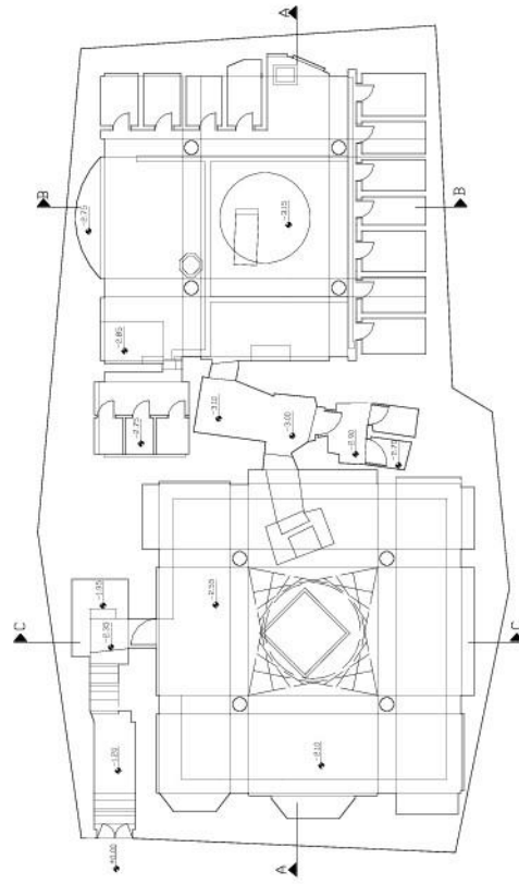
پلان حمام نظافت
