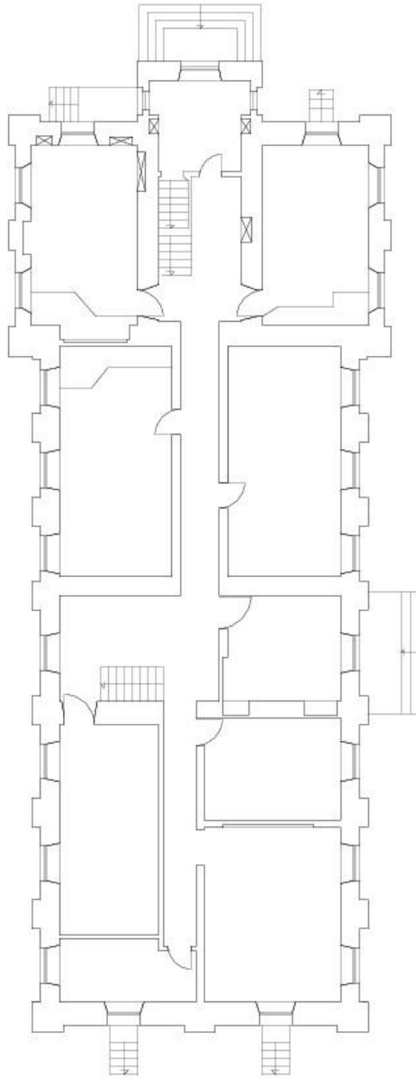
پلان طبقه اول
