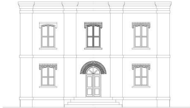
نمای غربی مدرسه
