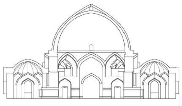
برش عرضی
